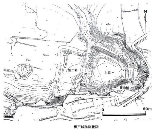
根戸城跡の測量図
